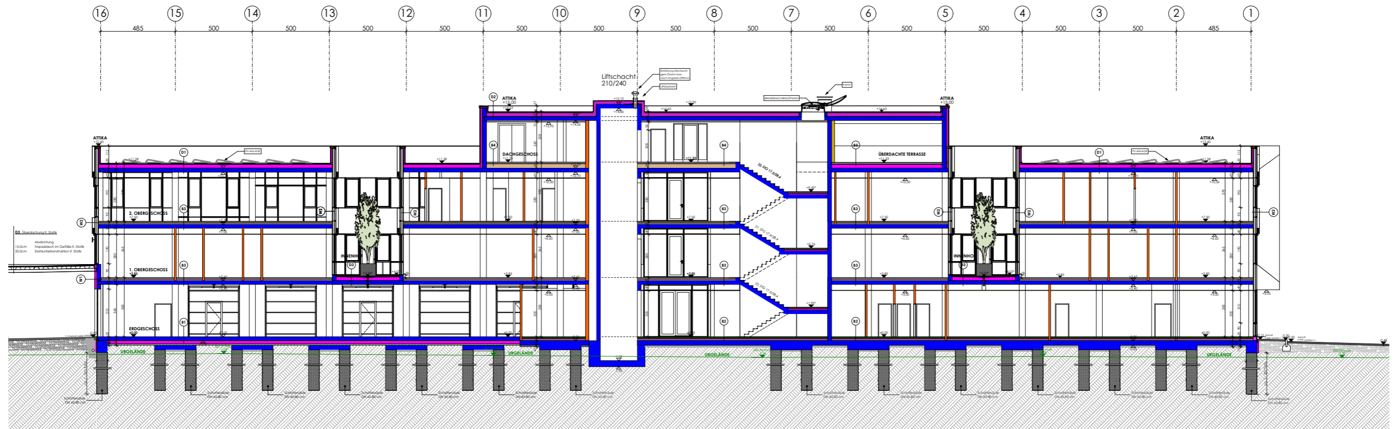
SCHNITT A:A
